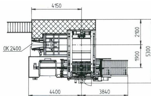
Vista en planta PIKOMAT HPS-Paletizador de sacos
