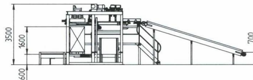
Vista lateral PIKOMAT HDQ - Compacto
