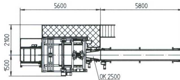
Вид сверху Pikommat HDQ Kompakt
