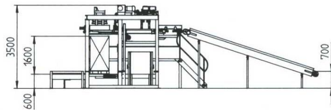
Вид со стороны Pikommat HDQ Kompakt
